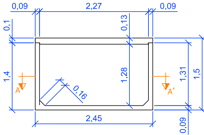
SECCIÓN B-B'
